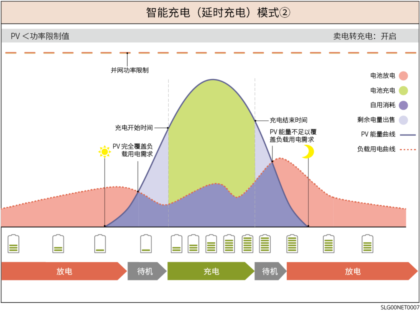
图7 智能充电（延时充电）模式2
