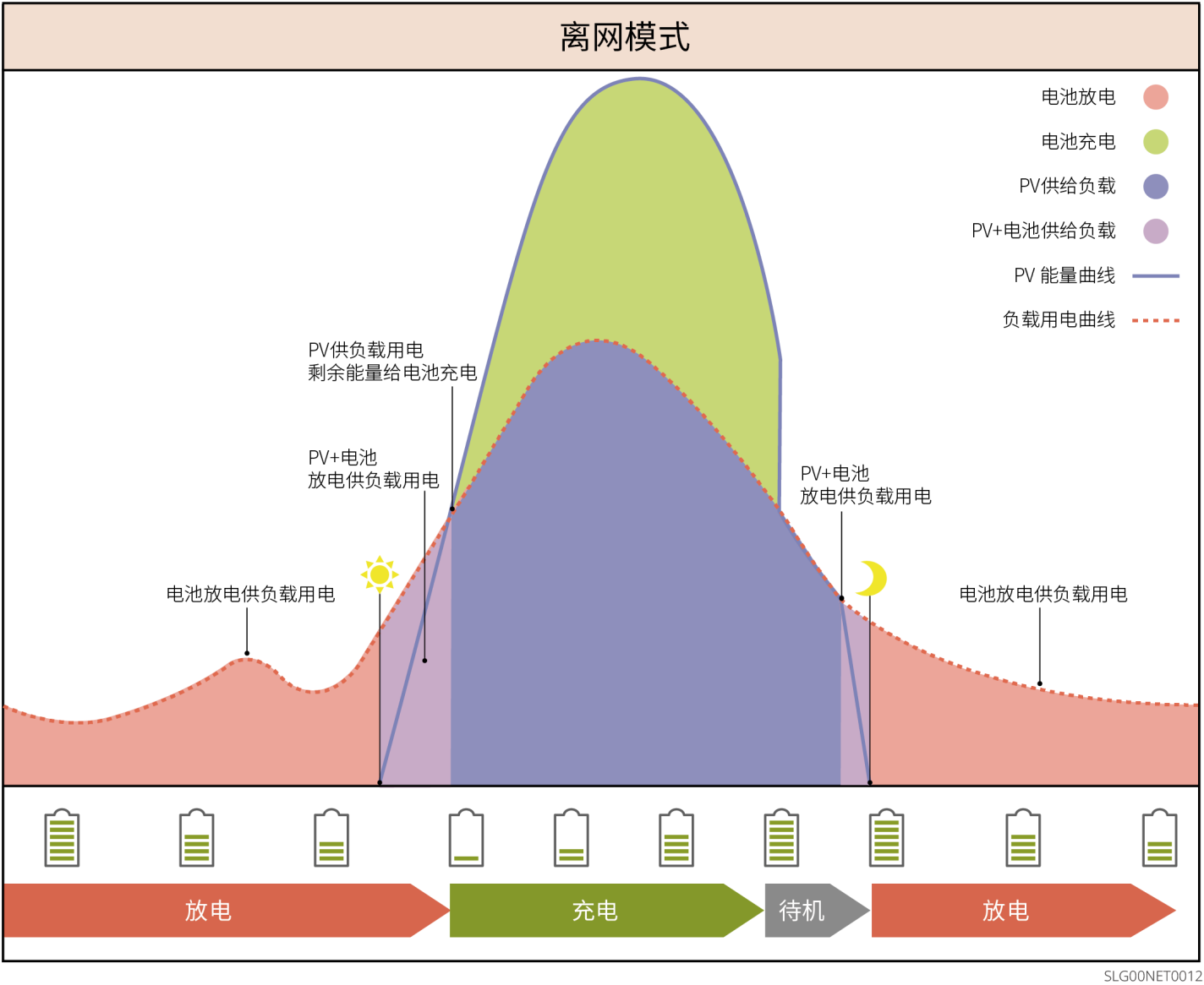
图10 离网模式
