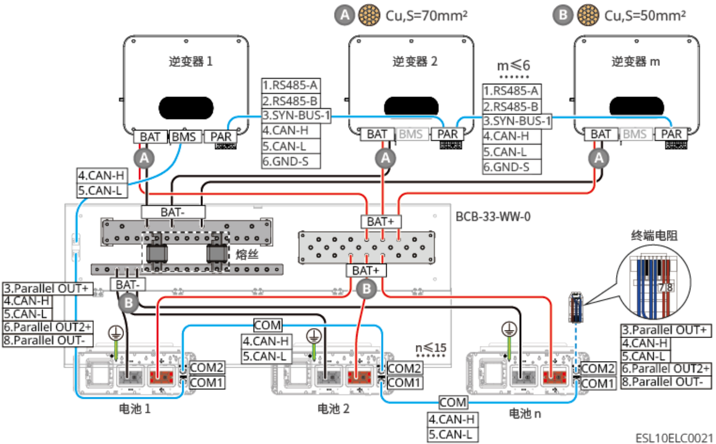
图27 LX U5.0-30：当电池数量 \leq 15 台，电池搭配汇流排BCB-33-WW-0连接方式
