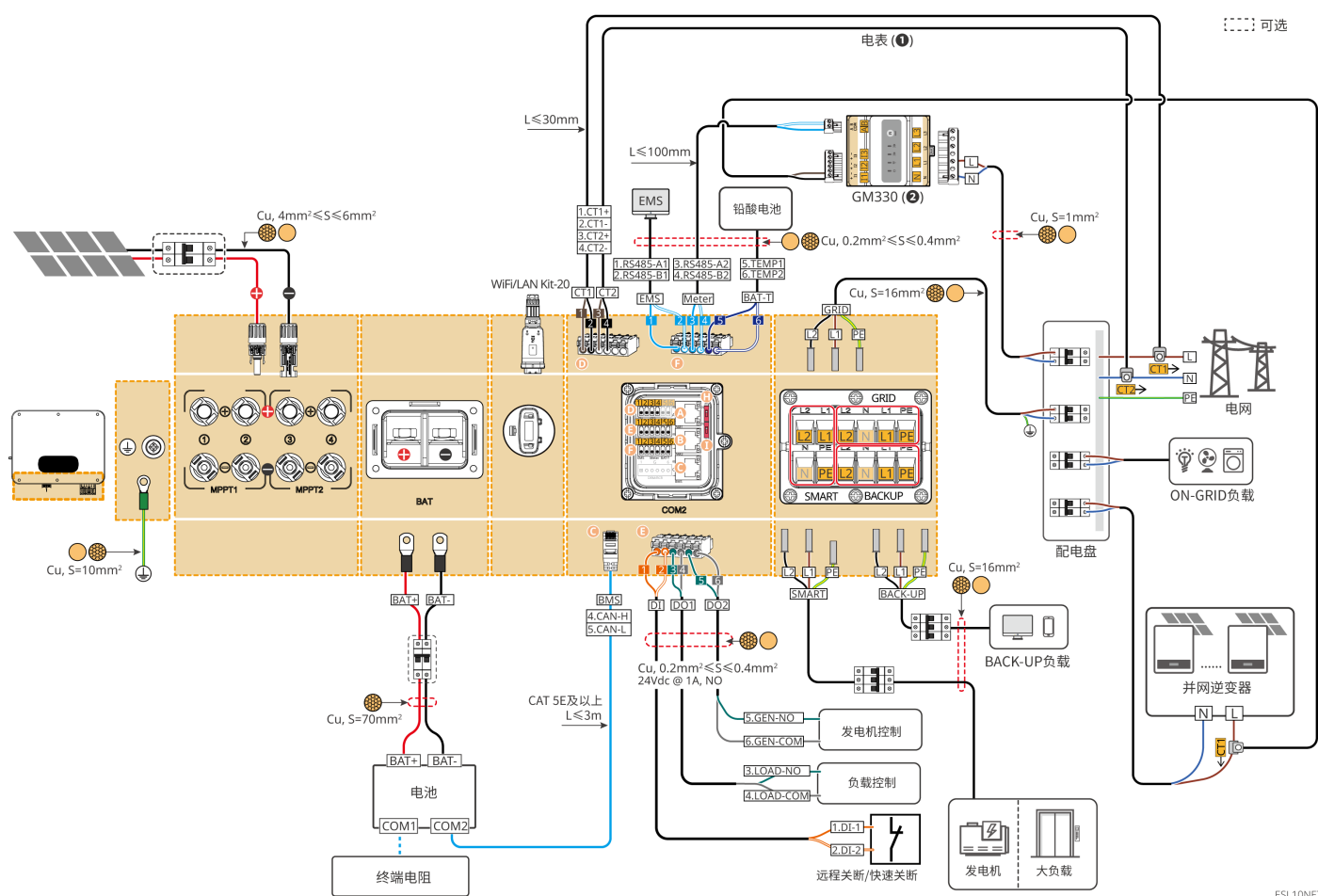
图13 耦合场景负载监控与并网机发电监测组网方案
