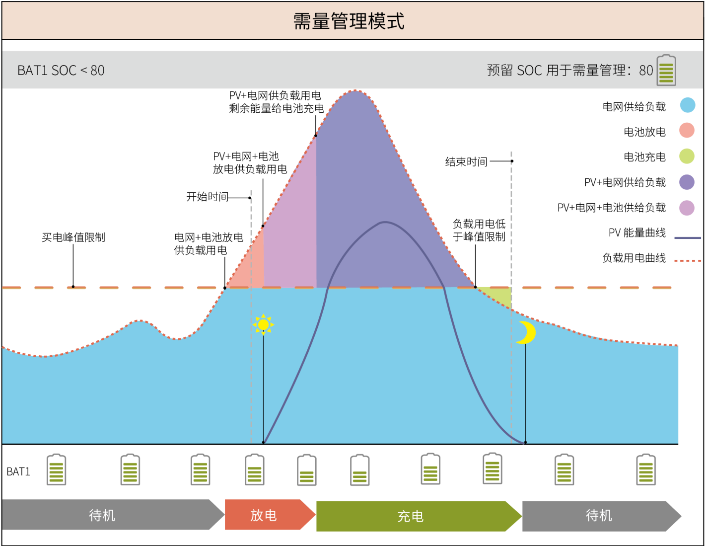
图9 需量管理模式
