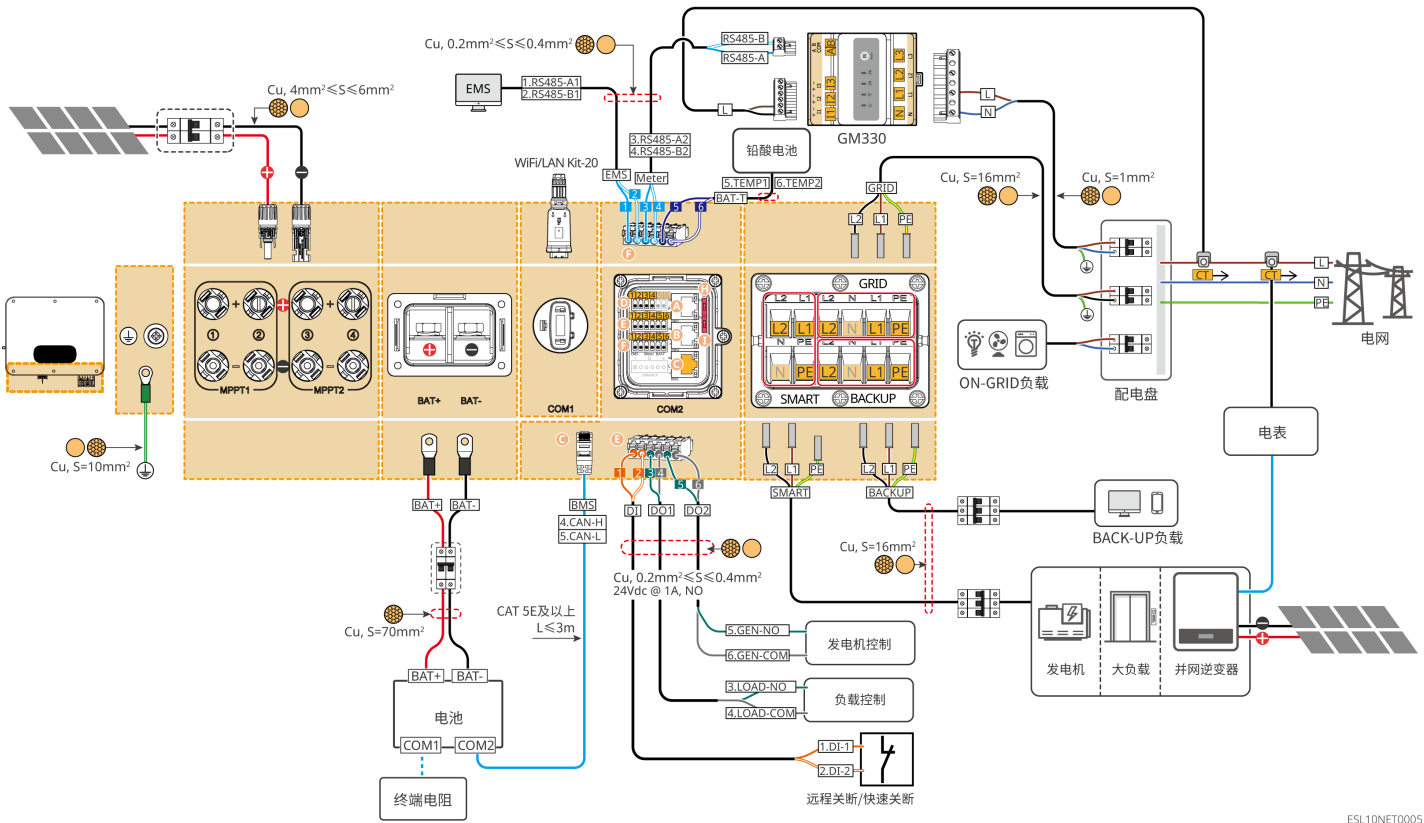
图12 搭配GM330场景
