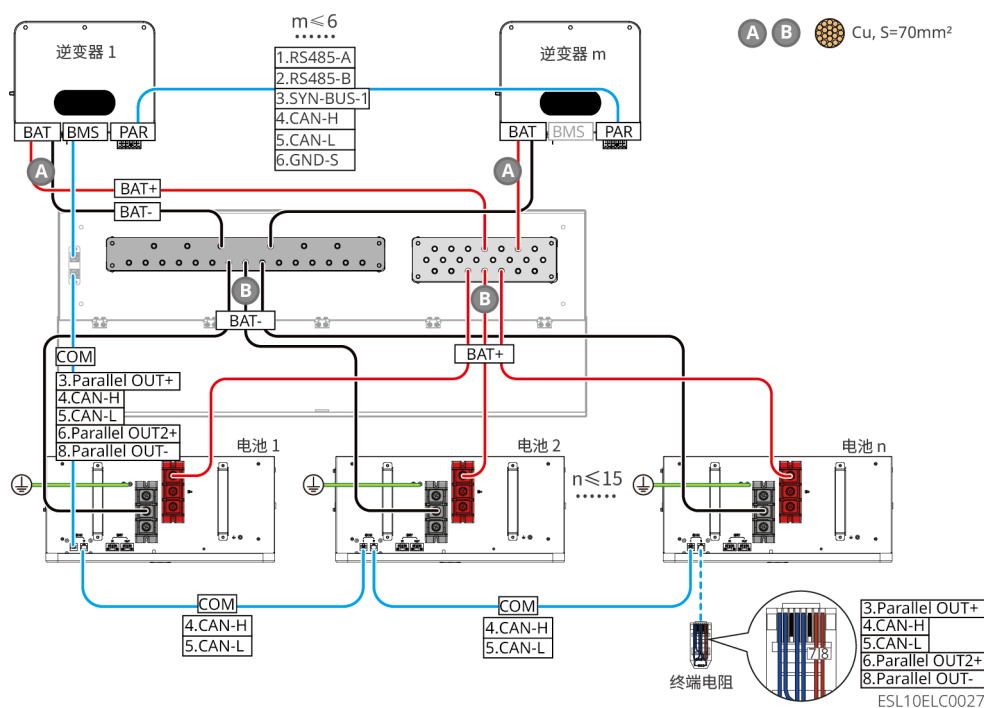
图32 GW14.3-BAT-LV-G10: 电池数量小于等于15, 使用汇流盒(BCB-32-WW-0, 电流 \leq 720\text{A} )连接1路输出逆变器
