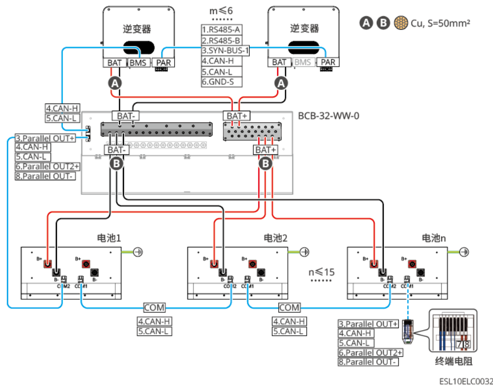
图34 GW16.1-BAT-LV-G10：电池数量小于等于15，使用汇流盒(BCB-32-WW-0, 电流 \leq 720A )连接逆变器
