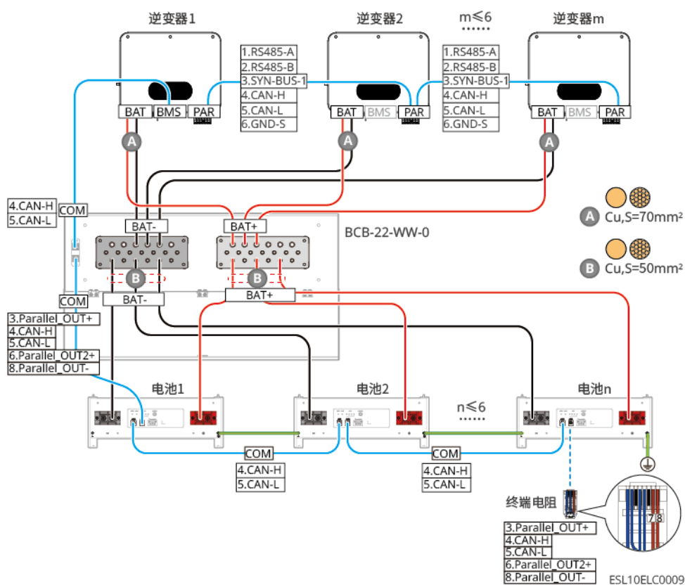
图22 LX A5.0-30：配合汇流盒BCB-22-WW-0连接方式
