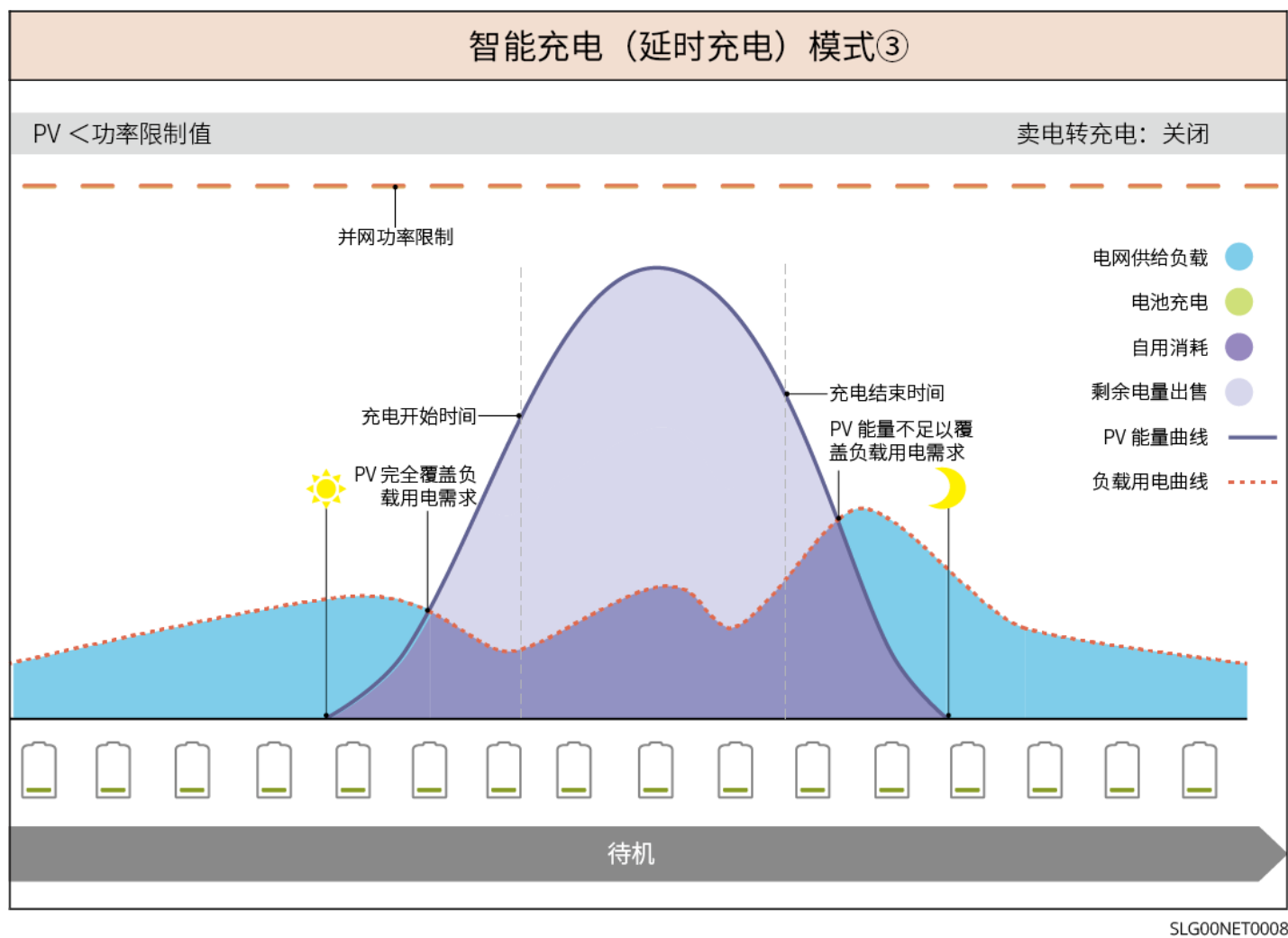
图8 智能充电（延时充电）模式3
