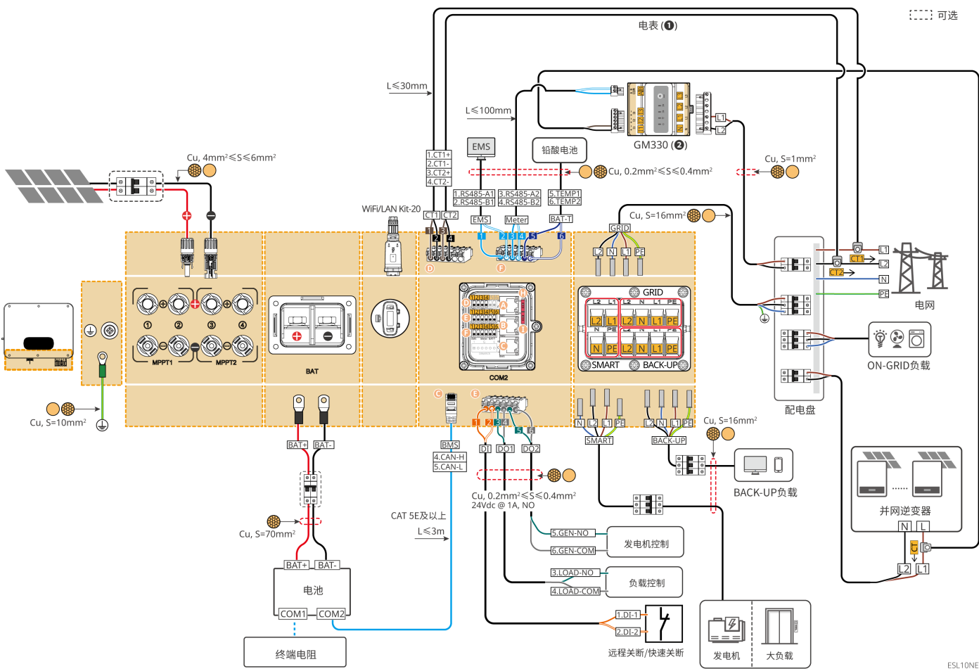
图16 耦合场景（接220V电网电压）
