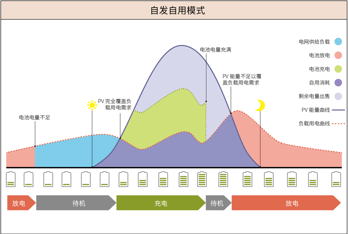
图1 自用模式
