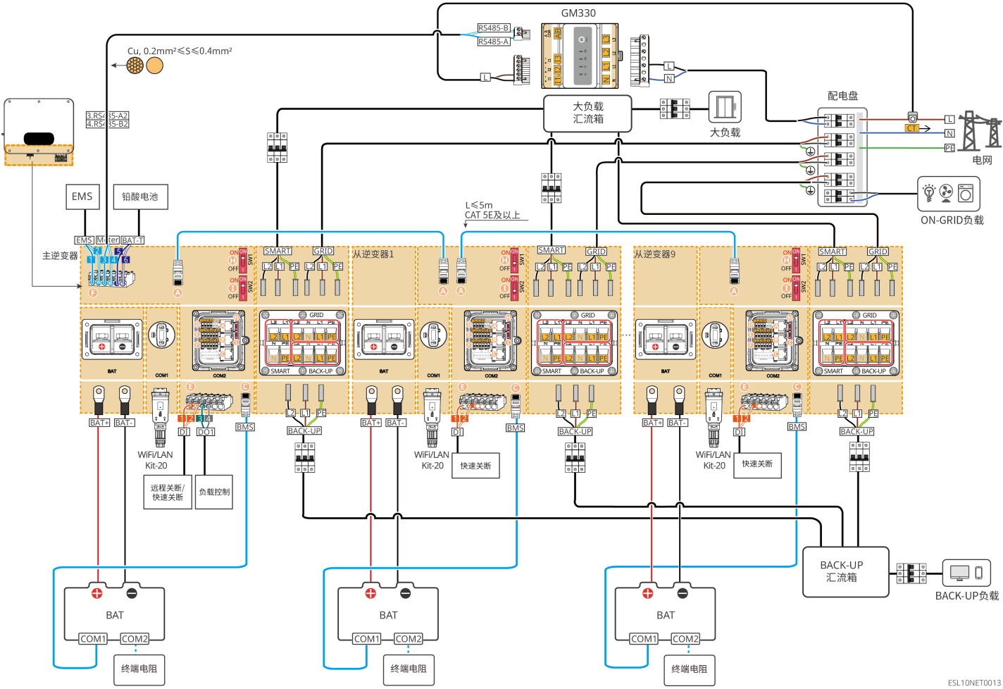
图18 搭配GM330场景
