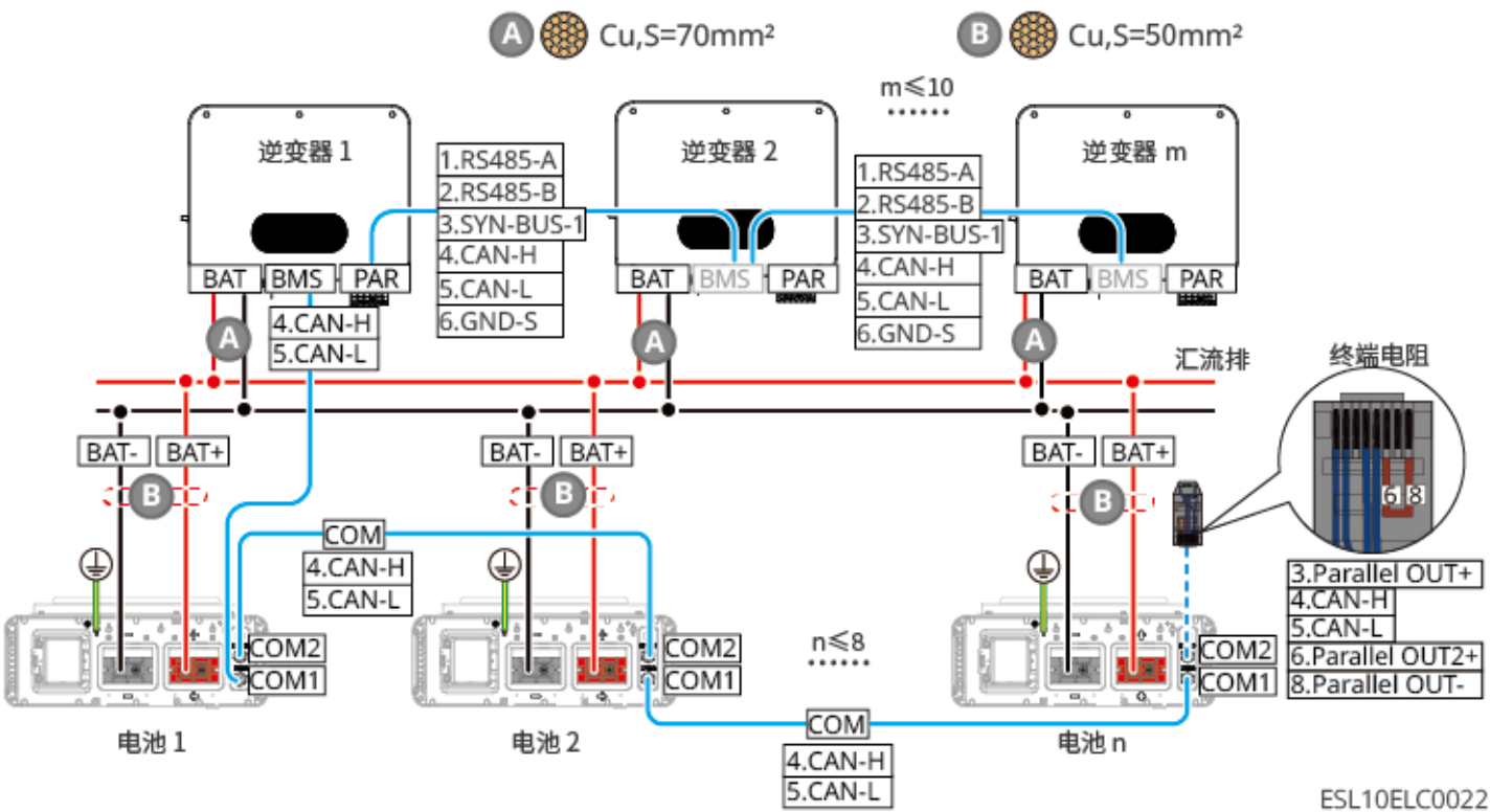
图28 LX U5.0-30: 当电池数量 \leq 8 台，电池搭配第三方汇流排连接方式
