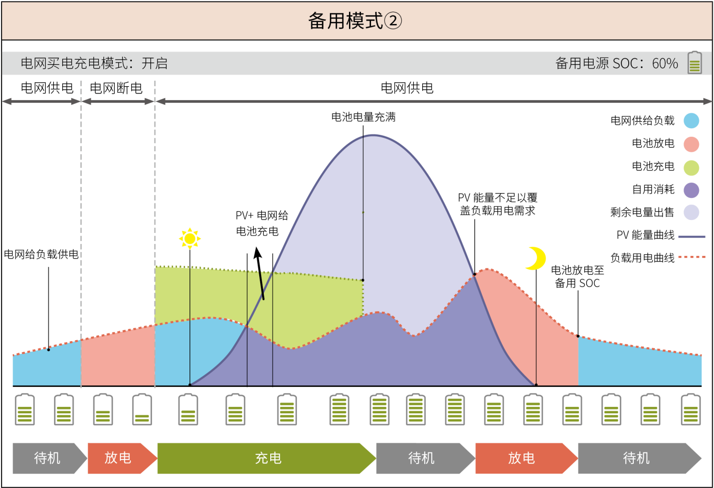
图3 备用模式2
