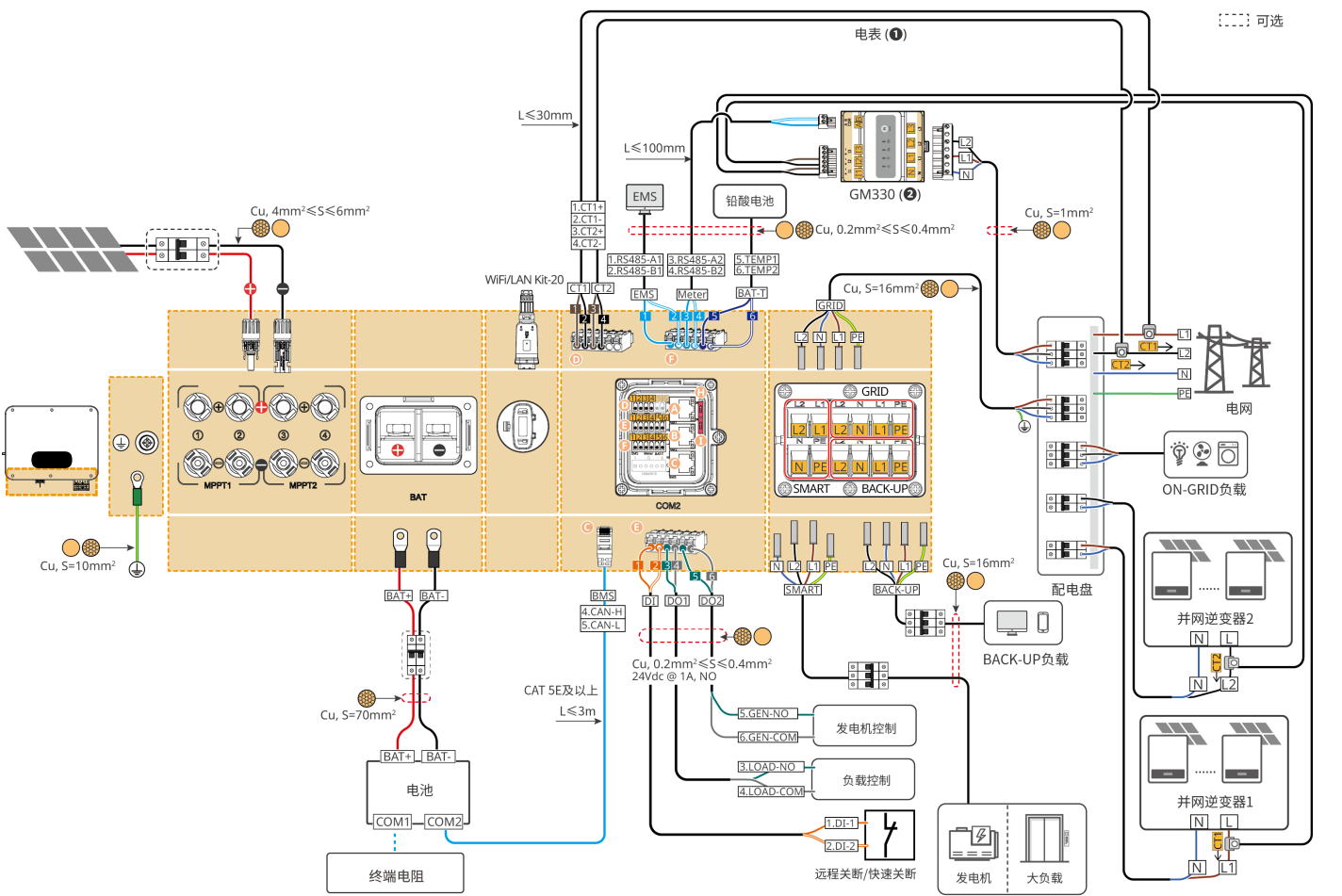
图15 耦合场景（接12V电网电压）
