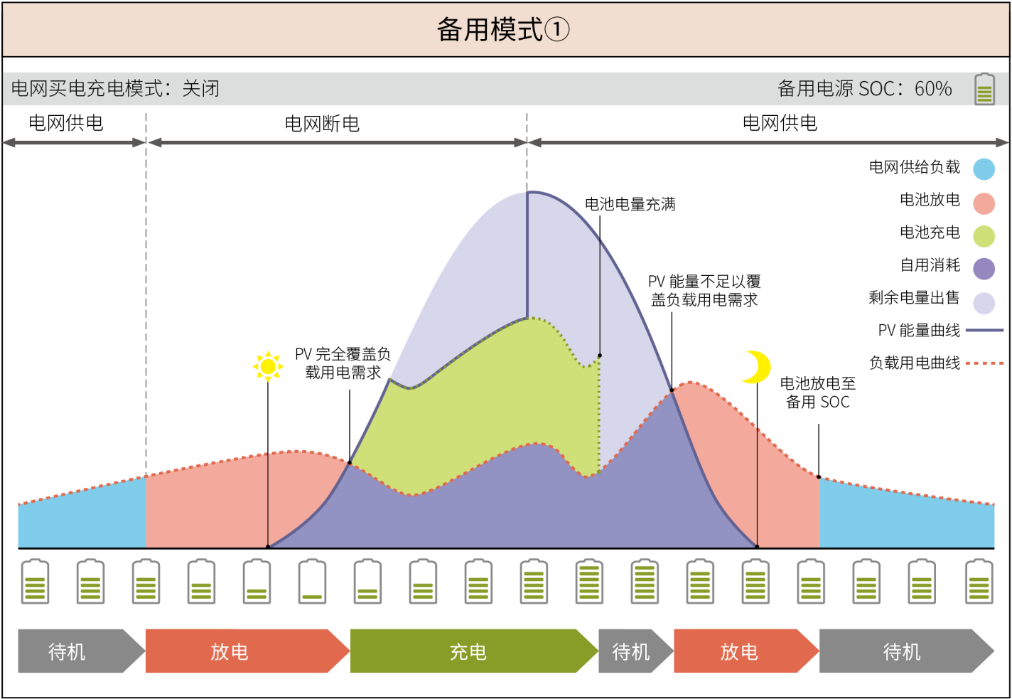
图2 备用模式1
