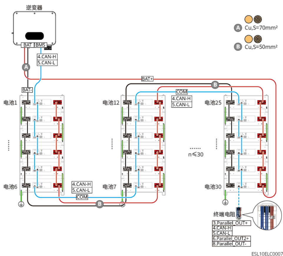
图21 LX A5.0-30: 手拉手连接方式
