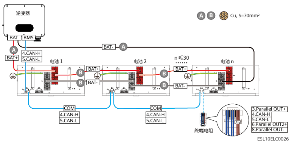
图31 GW14.3-BAT-LV-G10: 电池手拉手连接单台1路输出逆变器
