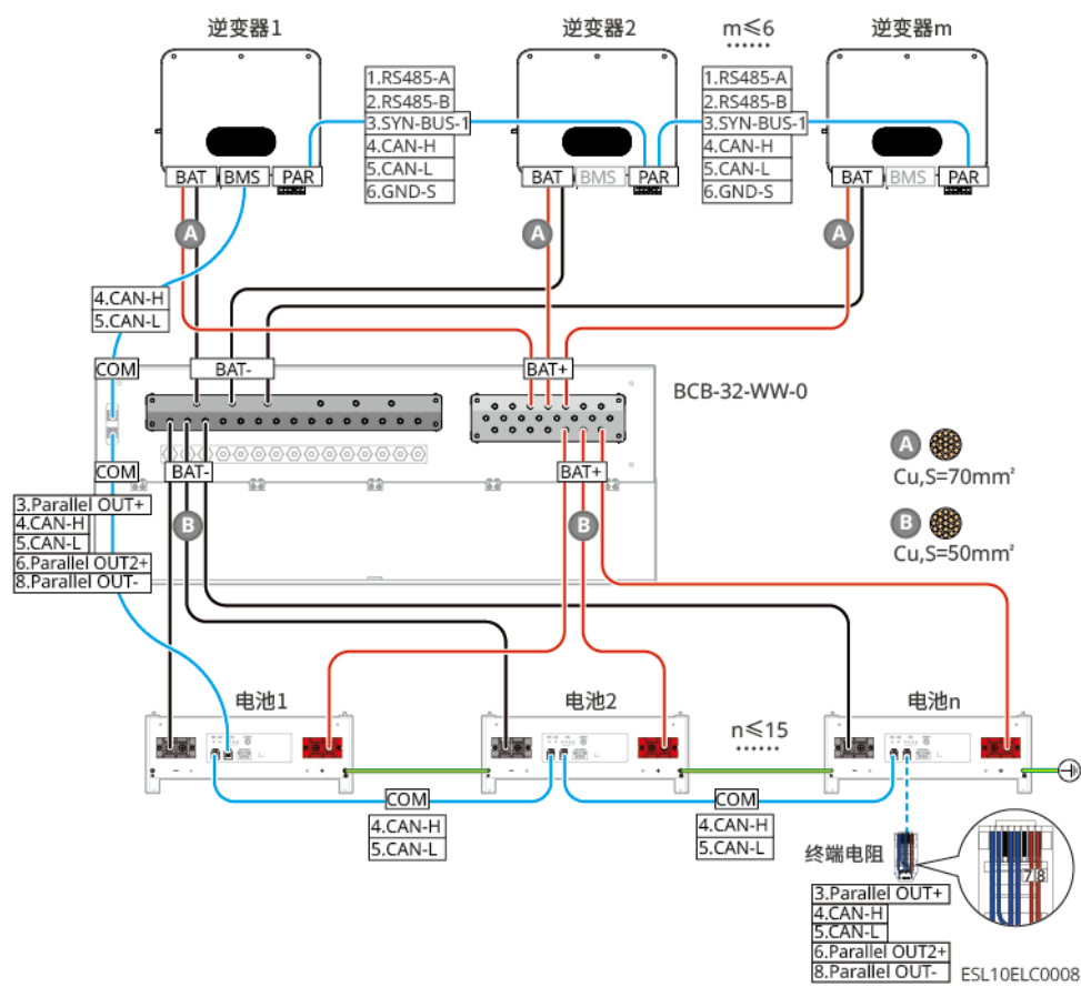
图23 LX A5.0-30：配合汇流盒BCB-32-WW-0连接方式
