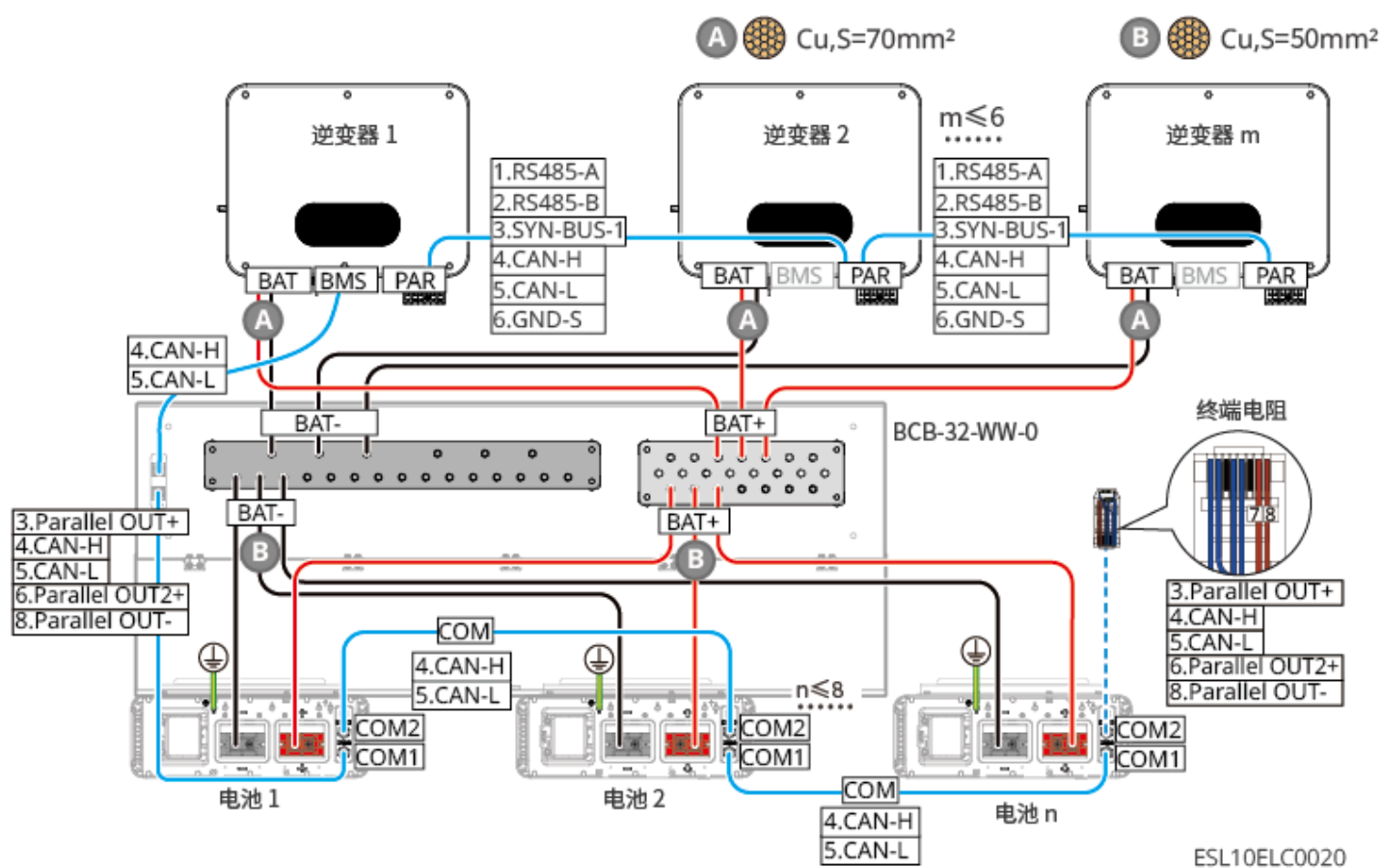
图26 LX U5.0-30: 当电池数量 \leq 8 台, 电池搭配BCB-32-WW-0连接方式
