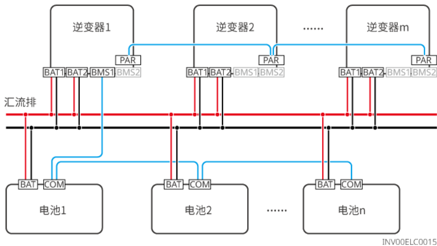
图35 逆变器并机时，电池配合第三方汇流排
