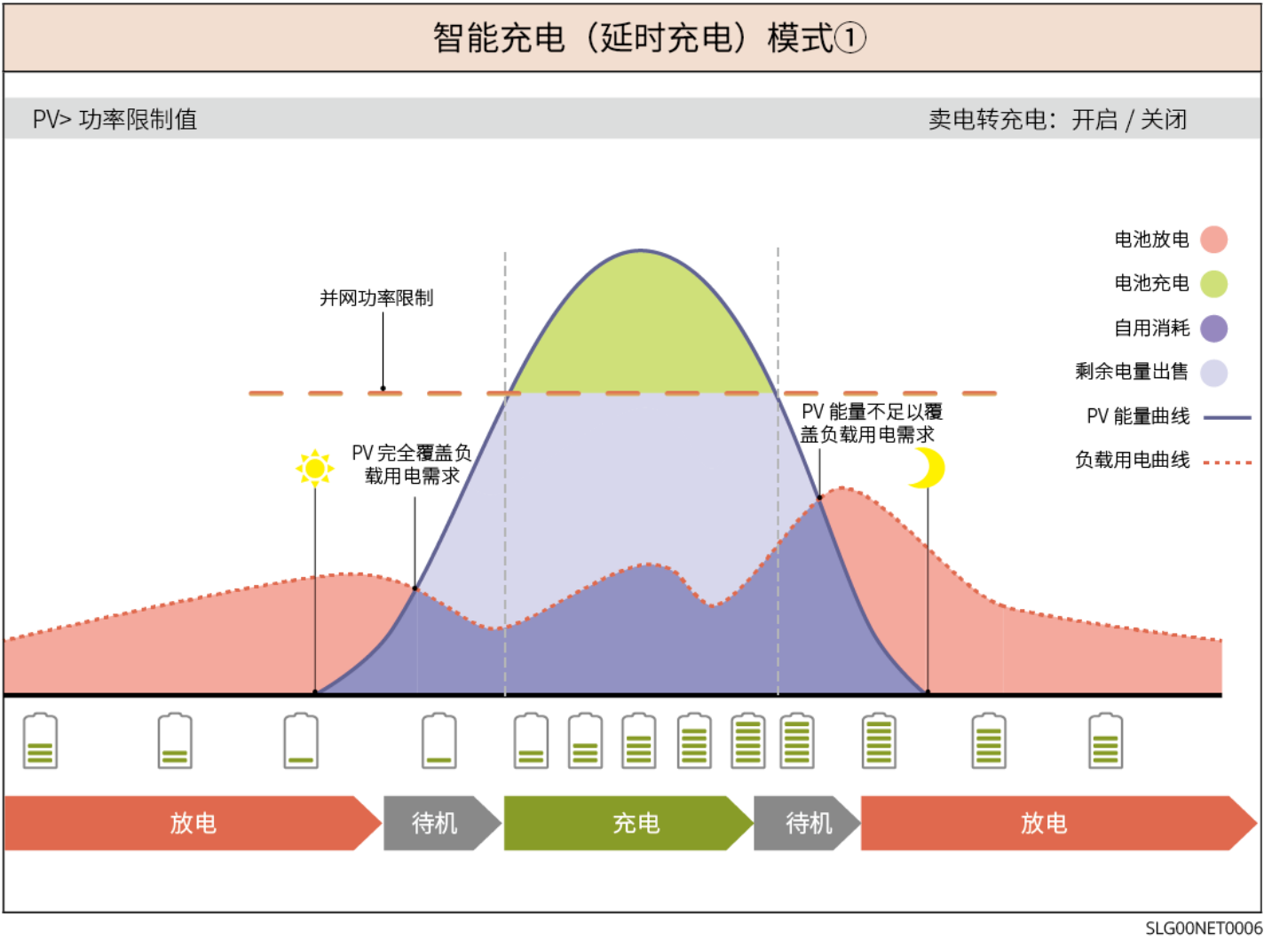
图6 智能充电（延时充电）模式1
