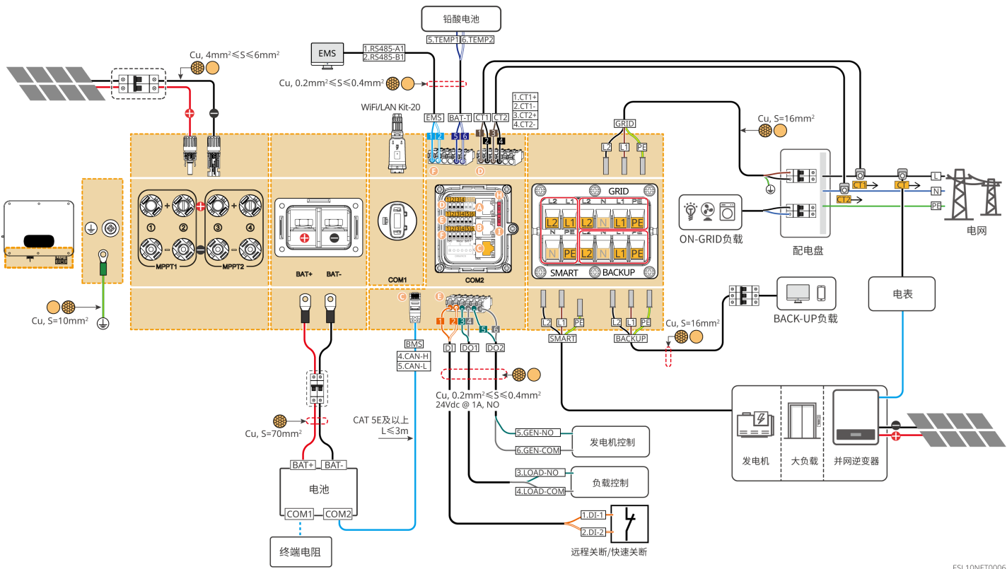
图11 搭配内置电表场景
