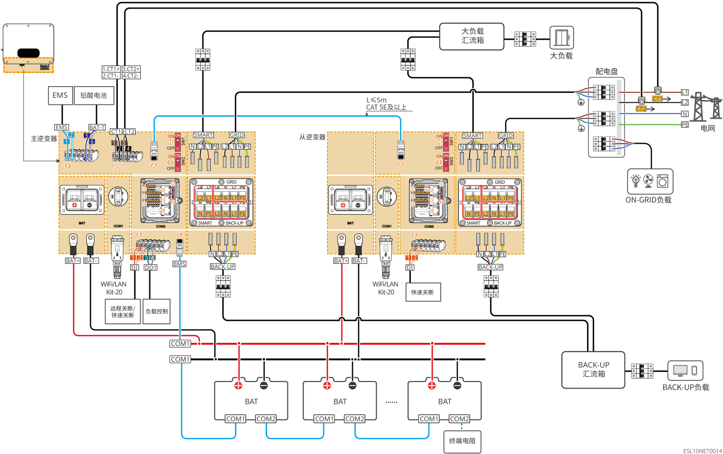
图19 搭配内置电表场景
