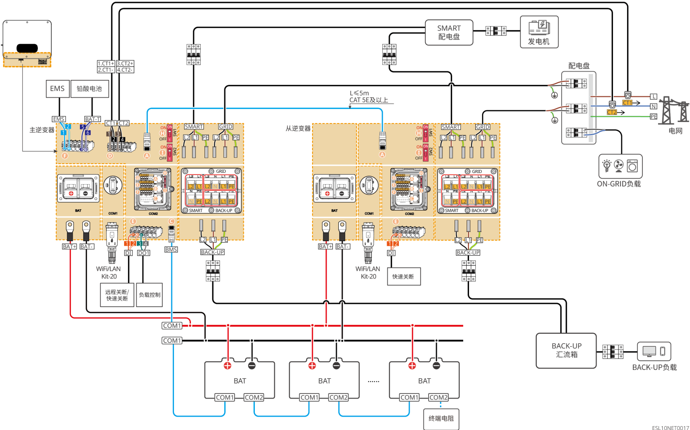
图17 搭配内置电表场景
