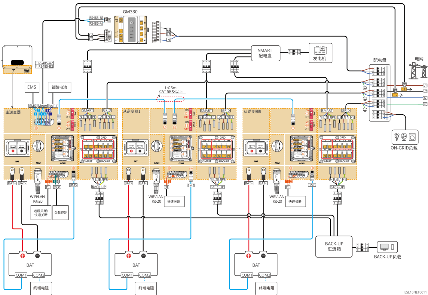
图20 搭配GM330场景
