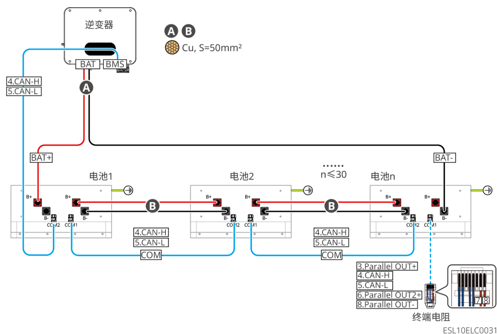
图33 GW16.1-BAT-LV-G10：电池手拉手连接逆变器
