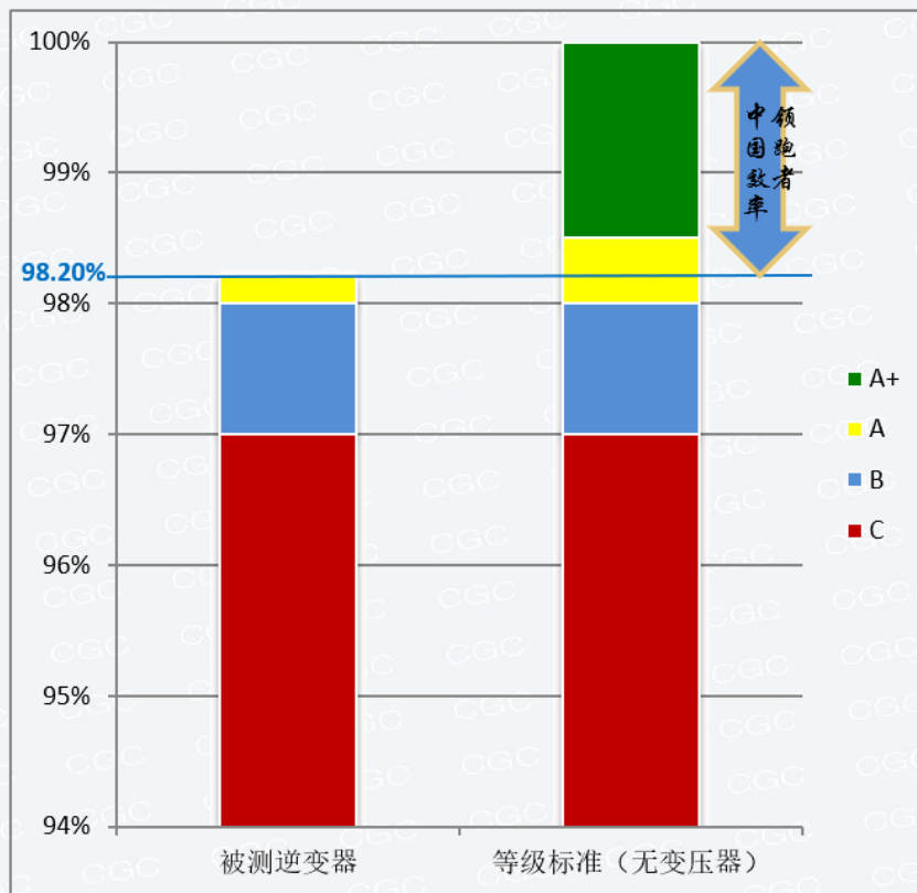
图 1. 逆变器效率水平对比图示
