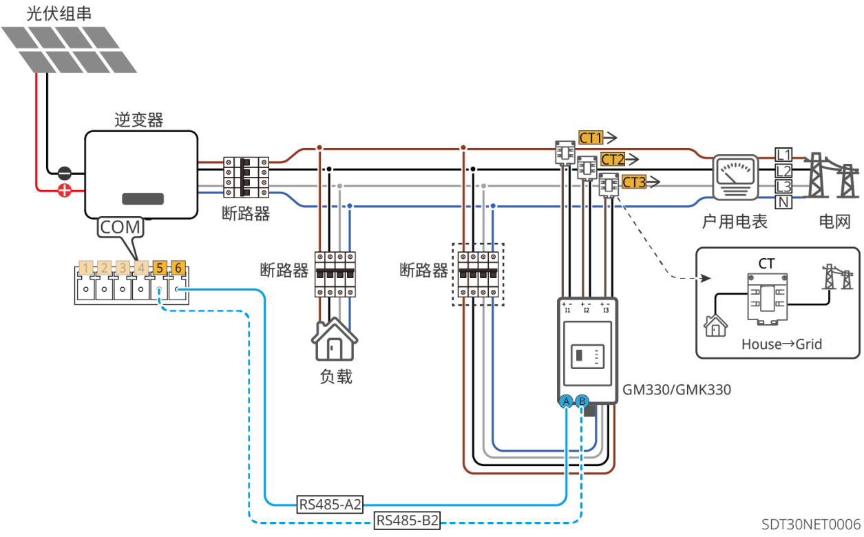
多机功率限制组网方案 (EzLogger Pro+GM330/GMK330)
