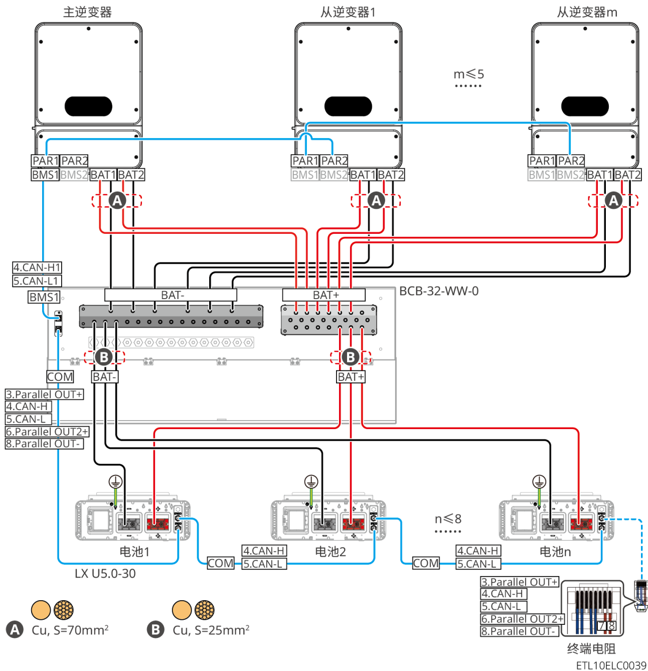
LX U5.0-30: 当电池数量 \leq 15 台，电池搭配汇流盒BCB-33-WW-0连接方式
