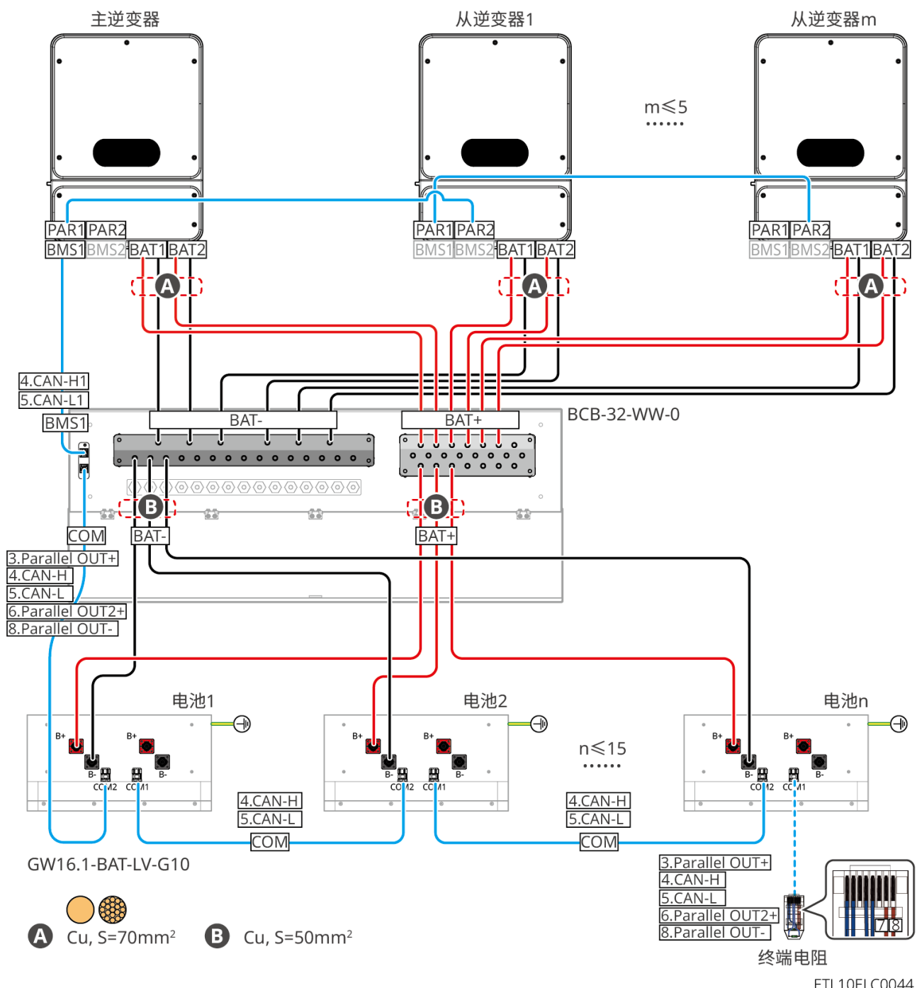
GW16.1-BAT-LV-G10：电池数量小于等于30，使用第三方汇流排接逆变器：
