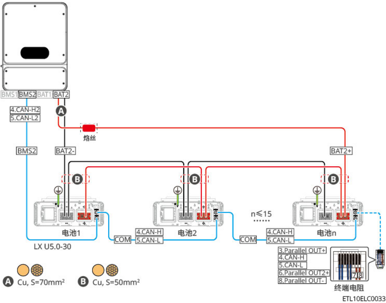
LX U5.0-30: 双路电池连接单台2路输出逆变器时
