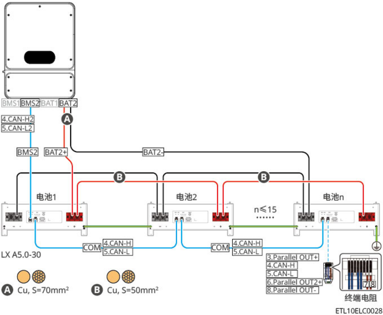
LX A5.0-30：两路电池连接单台2路输出逆变器时，接线图如下：
