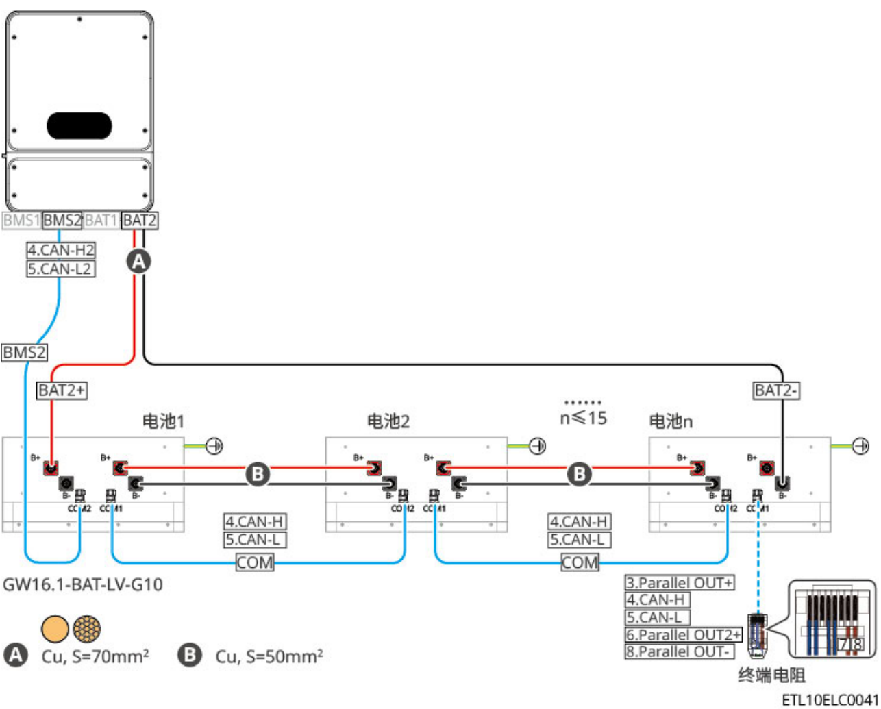
GW16.1-BAT-LV-G10：双路电池连接单台2路输出逆变器
