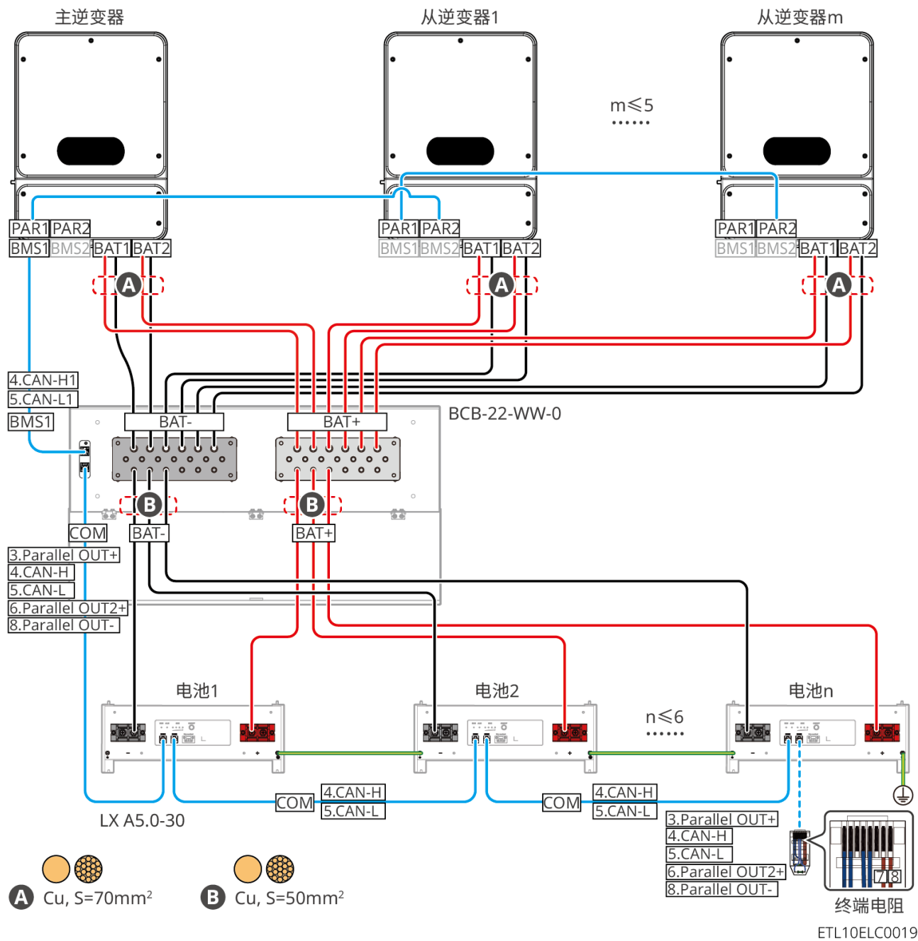
LX A5.0-30：配合汇流盒BCB-32-WW-0连接方式，接线图如下： 电池系统最大支持720A工作电流、36kW工作功率、最大连接6台逆变器、15台电池。
