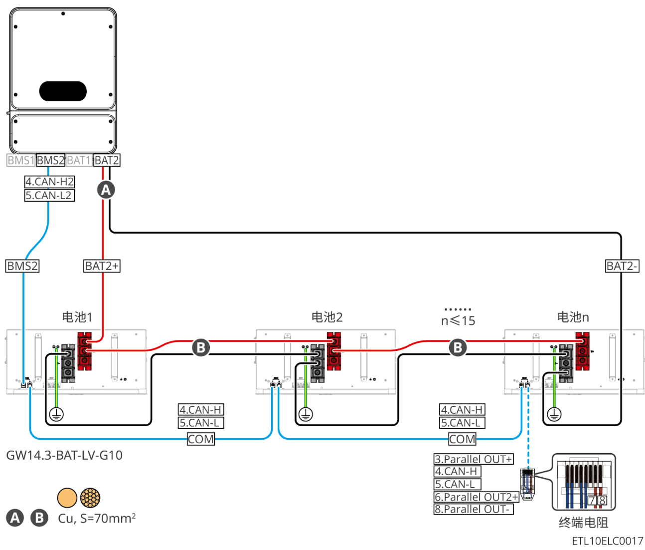
GW14.3-BAT-LV-G10：单路电池连接单台2路输出逆变器时 类型一：
