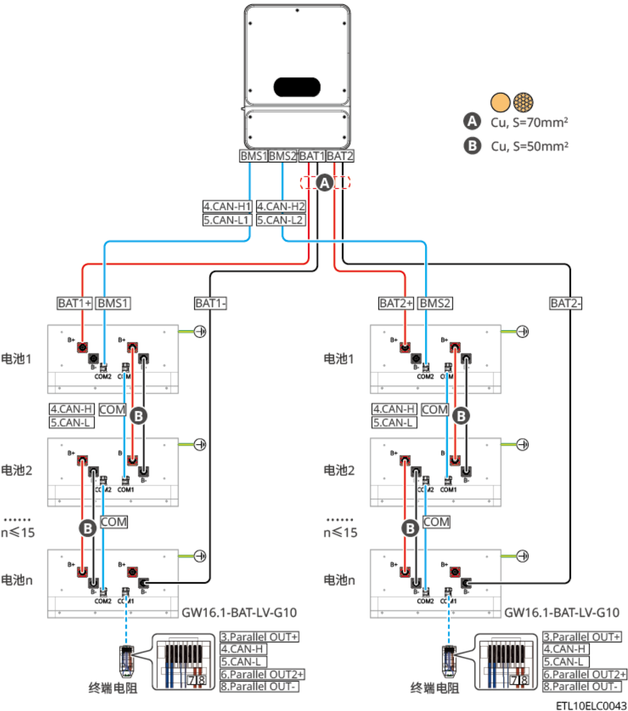
GW16.1-BAT-LV-G10： 电池数量小于等于15，使用汇流盒(BCB-32-WW-0, 电流≤720A)连接逆变器：
