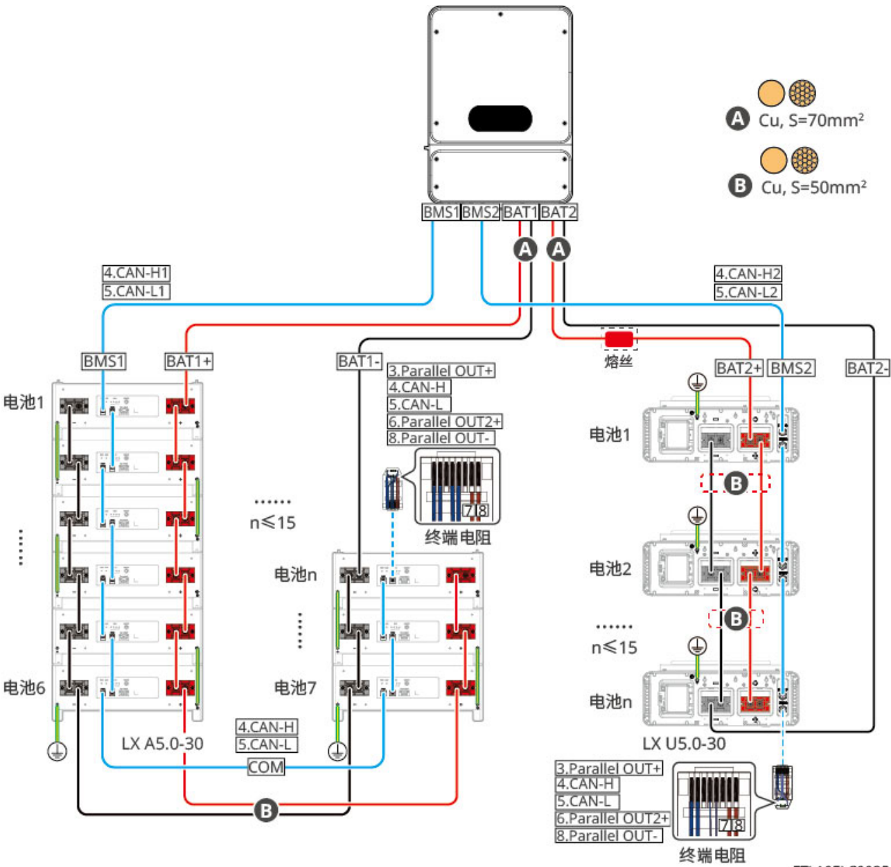
GW16.1-BAT-LV-G10： 单路电池连接单台2路输出逆变器 类型一：
