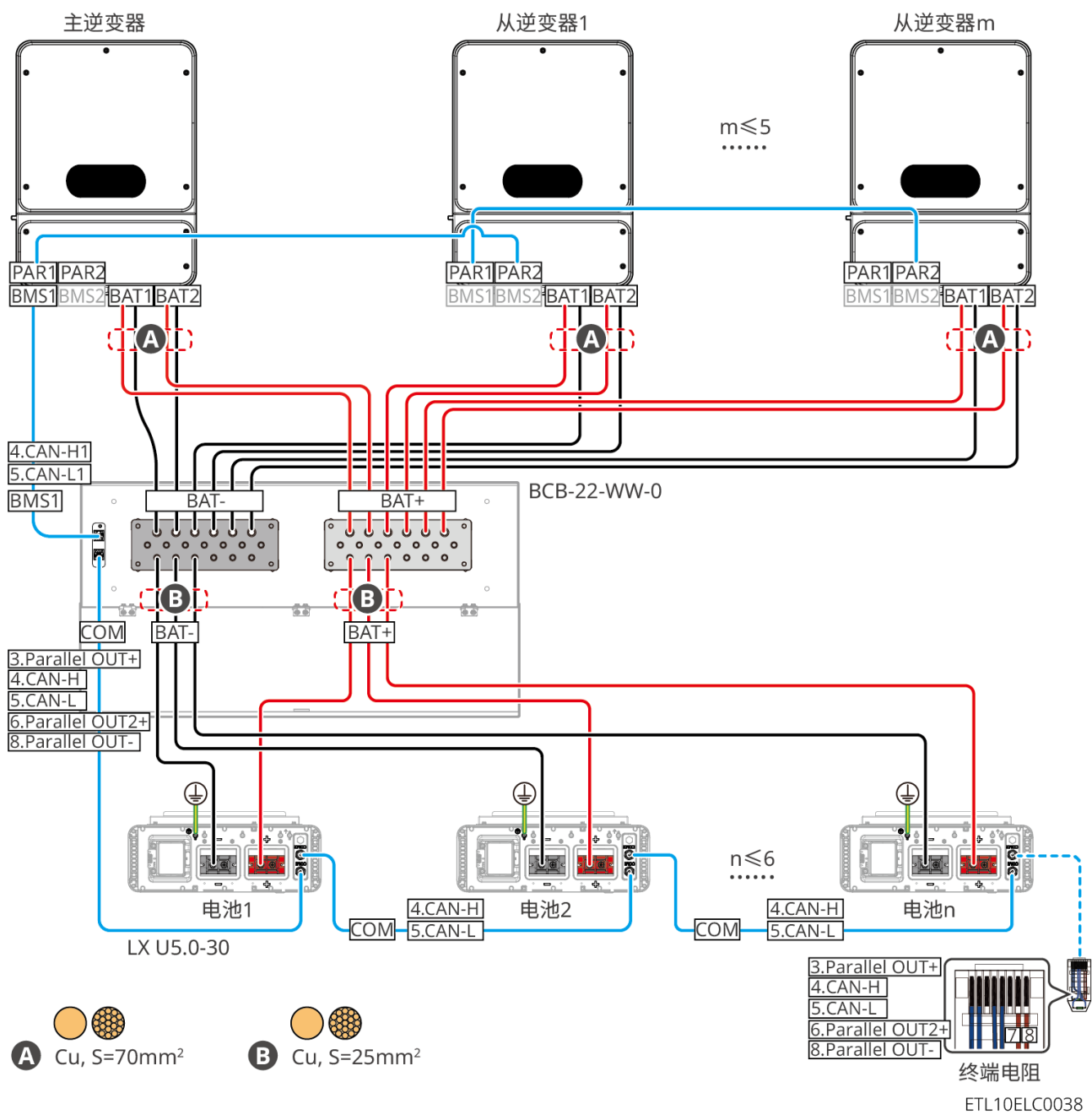
LX U5.0-30：当电池数量 \leq 8 台，电池搭配BCB-32-WW-0连接方式
