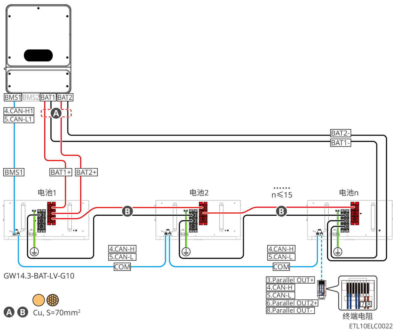
GW14.3-BAT-LV-G10：双路电池连接单台2路输出逆变器时
