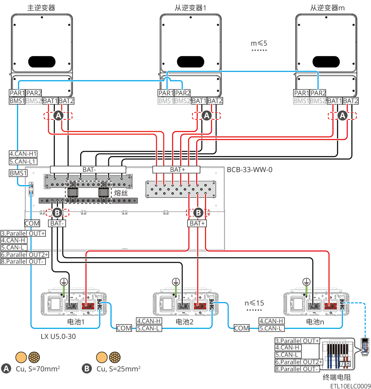
LX U5.0-30: 当电池数量 \leq 8 台，电池搭配第三方汇流排连接方式
