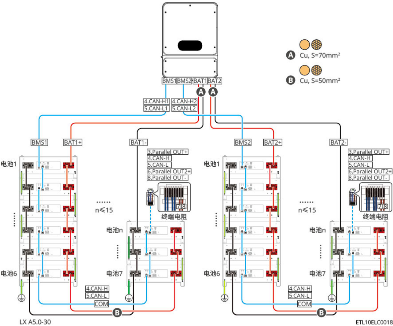
LXA5.0-30：配合汇流盒BCB-22-WW-0连接方式，接线图如下： 电池系统最大支持720A工作电流、36kW工作功率、最大连接6台逆变器、6台电池。
