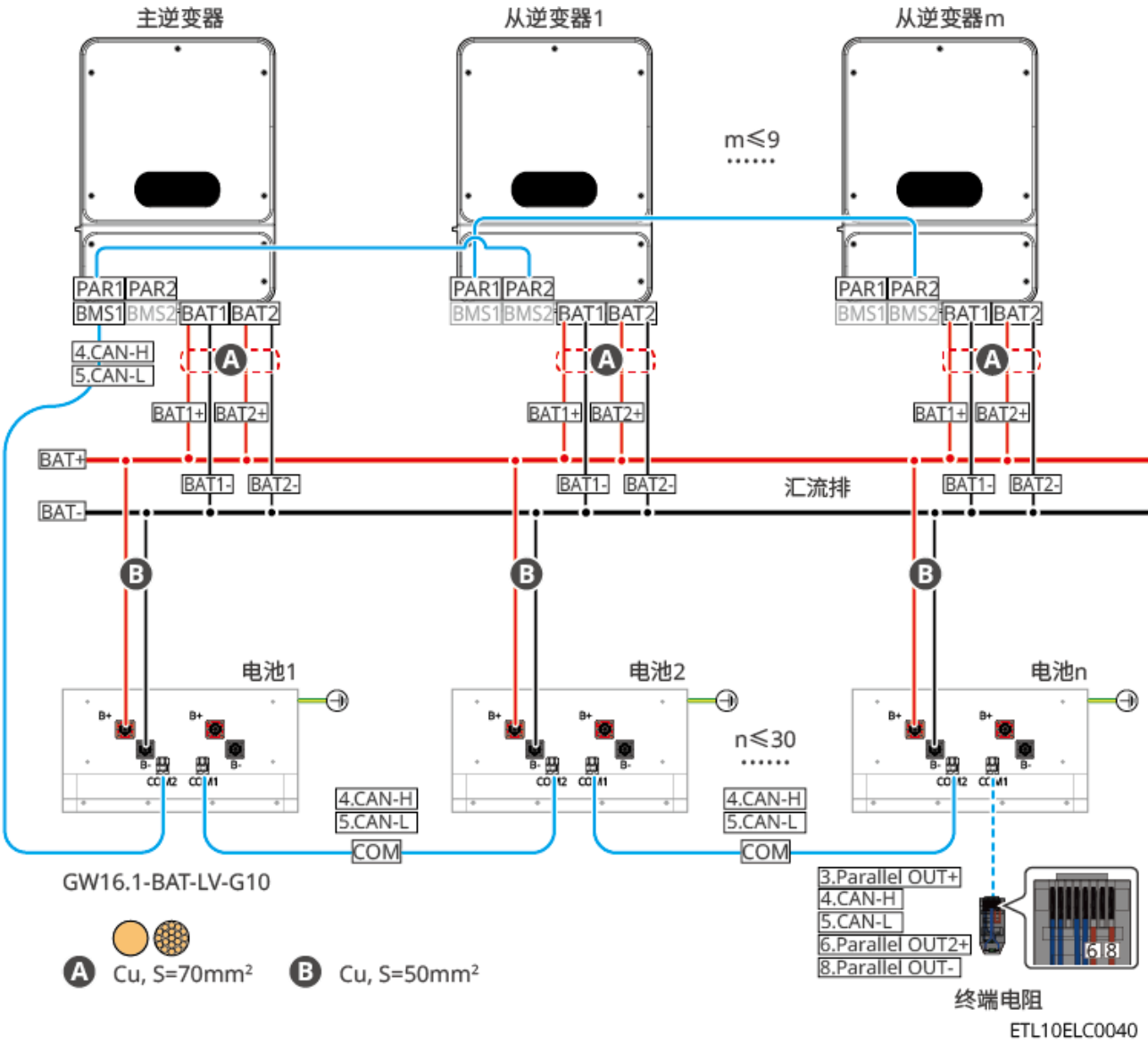
铅酸电池搭配汇流排连接方式
