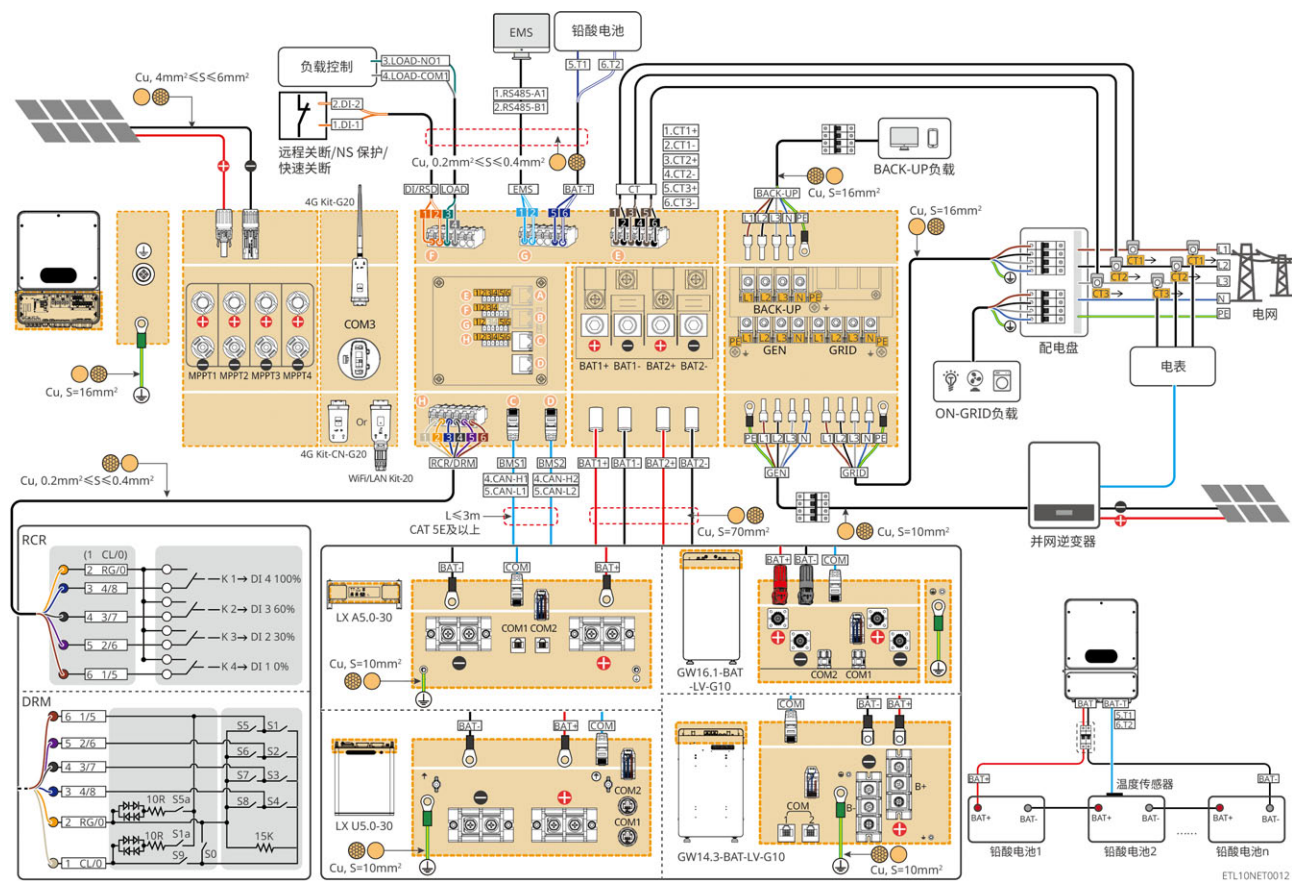
搭配GM330电表场景
