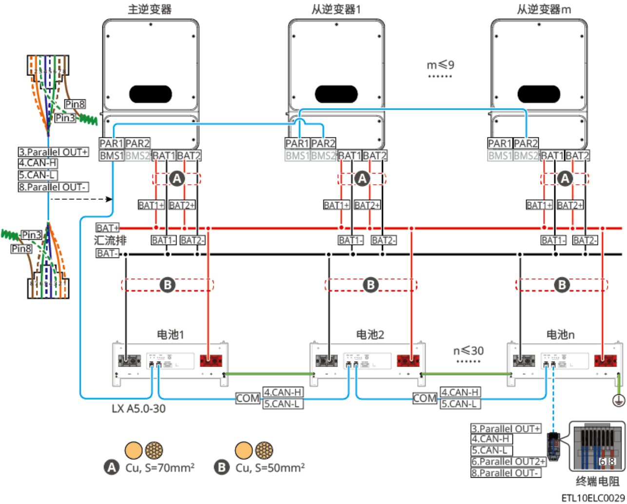
GW14.3-BAT-LV-G10：手拉手连接方式 电池连接单台2路输出逆变器时 类型一：
