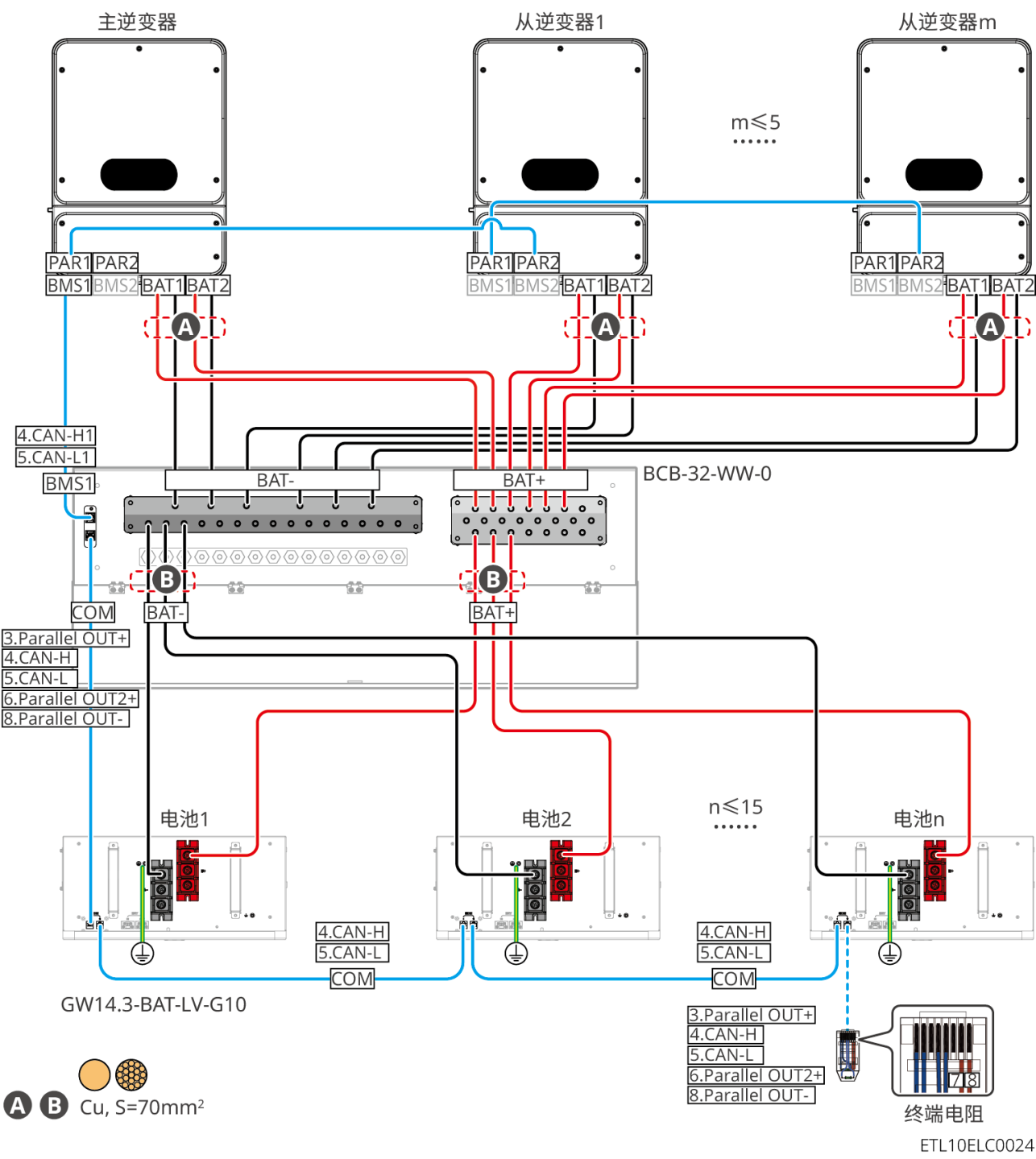
GW14.3-BAT-LV-G10：配合第三方汇流排连接方式
